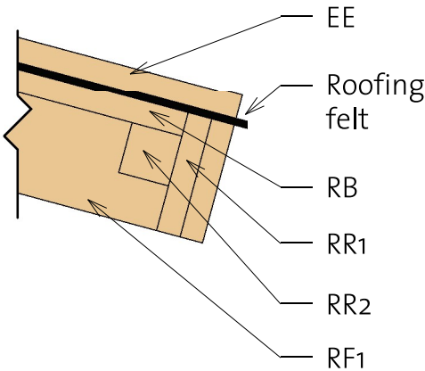
2 Facia
